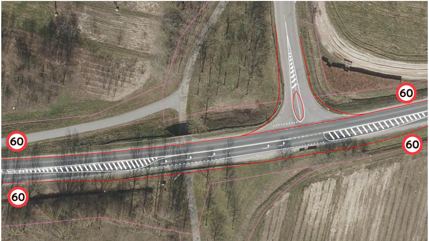
Princip for krydsudvidelse med ny venstresvingbane og sekundærhelle.
